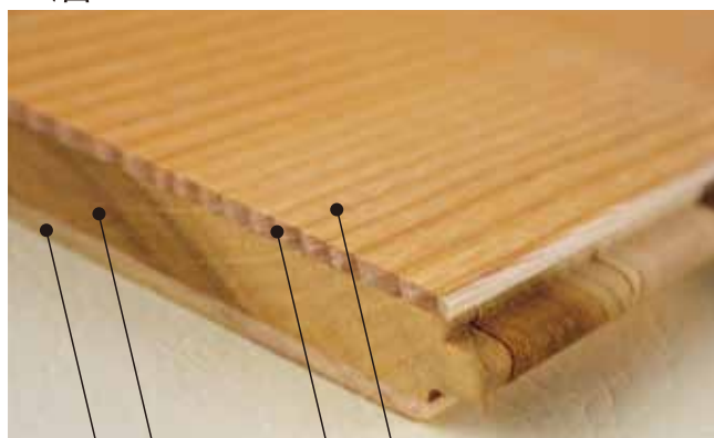
天然木 9mm 天然木 3mm 植物オイル・UV塗料（無塗装可） 単板 3mm
